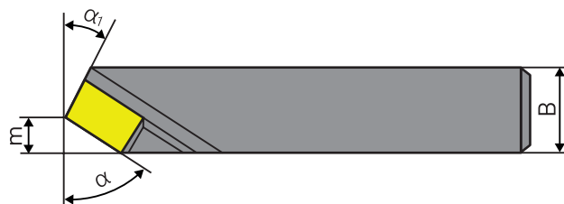
Левый резец
