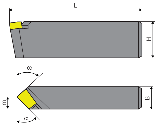
Левый резец
