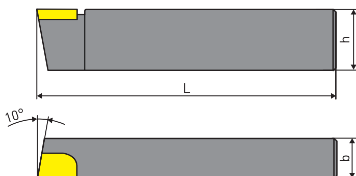
Левый резец
