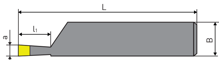
Левый резец
